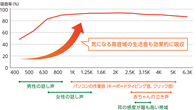
〈残響室法吸音率〉※残響室にて測定
